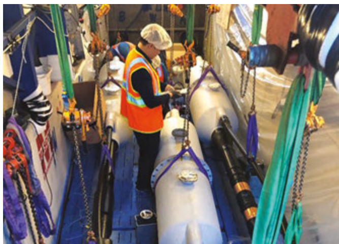
وصل واختبار أجزاء الكابلات وداخل حوض التوصيلات في Rawson Road, Greenacre
